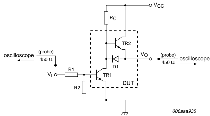
I_C = 0.05\text{ A} ; I_B = 2.5\text{ mA} ; R_1 = 1\text{ k}\Omega ; R_2 = 1\text{ k}\Omega ; R_C = 180\text{ }\Omega
